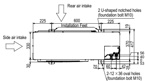
Außengeräte Zubadan Inverter, PUHZ-HRP200YKA
