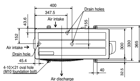
Außengeräte Power Inverter, PUHZ-RP35/50VHA
