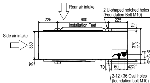
Außengeräte Power Inverter, PUHZ-RP100-140 YKA
